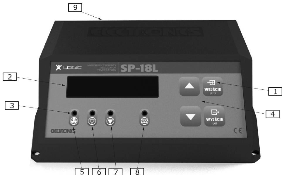
Widok regulatora wraz z zaznaczonymi funkcjami
